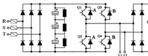
Схема инверторного модуля
